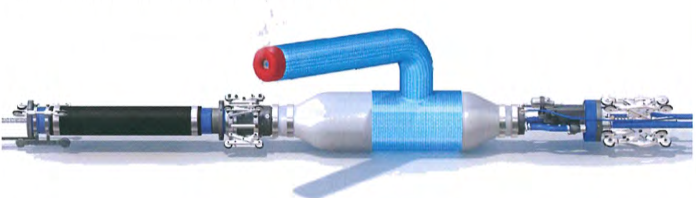
D. Voll aufgeblasener DrainMtH-Liner mit LinerEndCap
