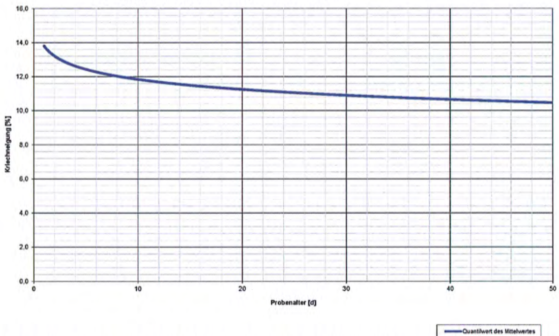
Diagramm 3: "Beurteilung der Kriechneigung in Abhängigkeit des Probenalters des Harzsystems "epros®EPROPOX HC120+""
