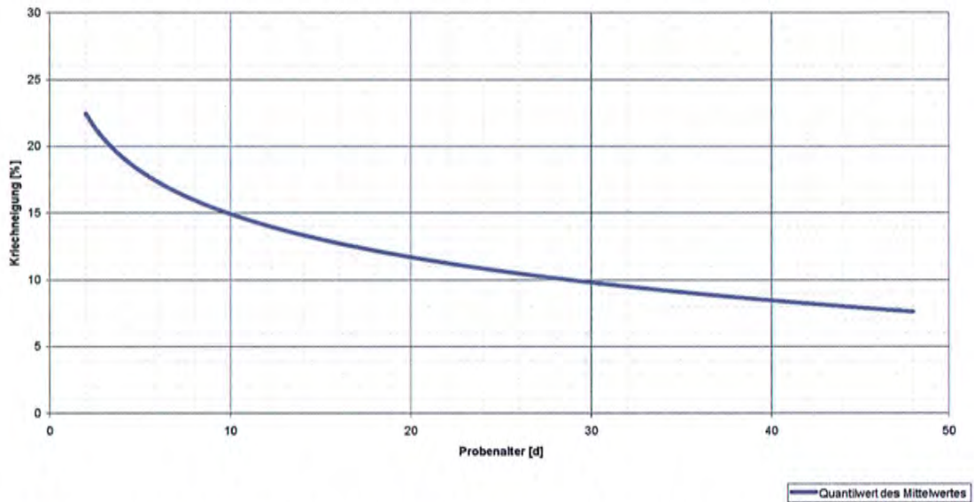
Diagramm 3: "Beurteilung der Kriechneigung in Abhängigkeit des Probenalters des Harzsystems "epros®EPROPOX HC120+""
