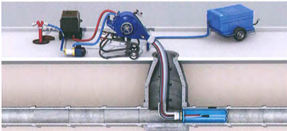
2. Inversion des Schlauchliners, Heizschlauch wird mit inversiert.
