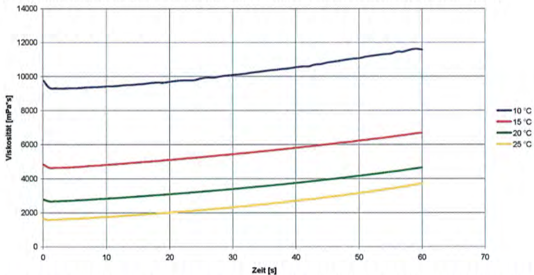
Diagramm 1: Mischungsviskosität des Harzsystems "epros®EPROPOX HC120+ (A+B)"
