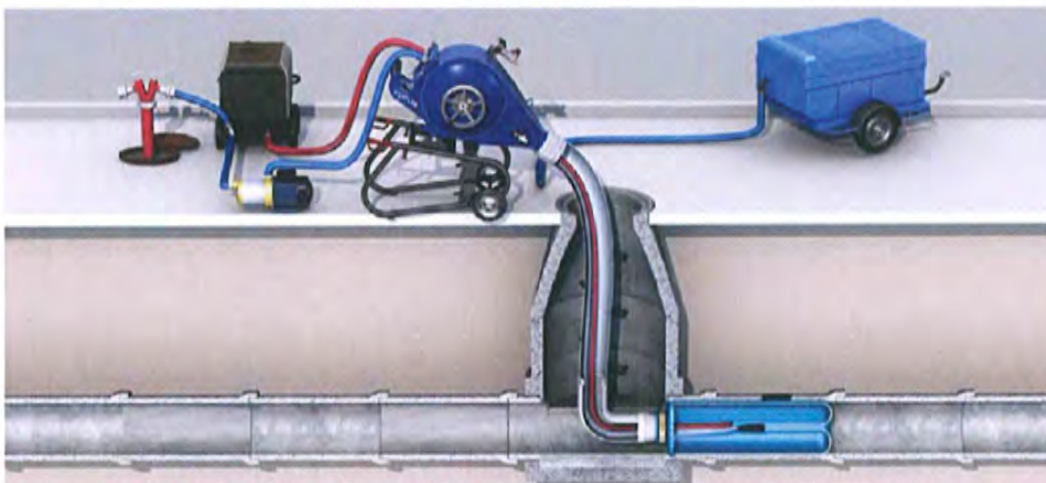
2. Inversion des Schlauchliners, Heizschlauch wird mit inversiert.
