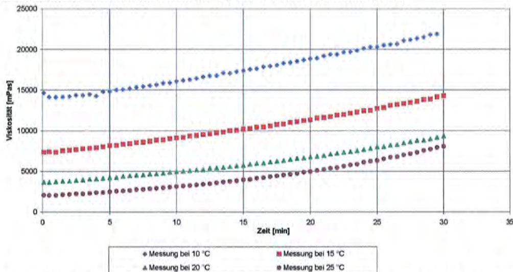
Diagramm 1: "Mischungsviskosität "epros®EPROPOX FC30 (A+B)""
